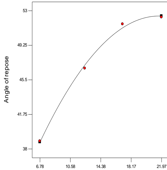
A: Moisture content
