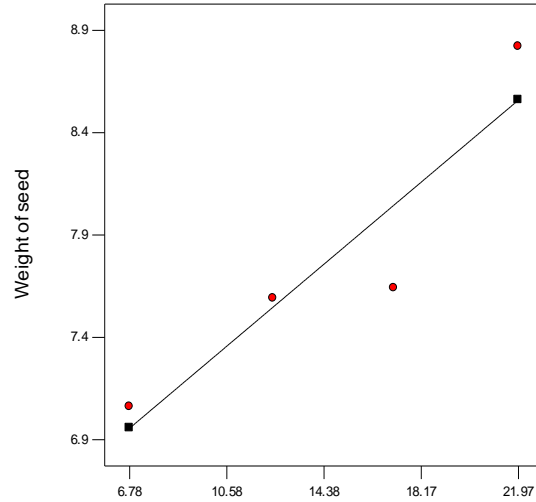
A: Moisture content
